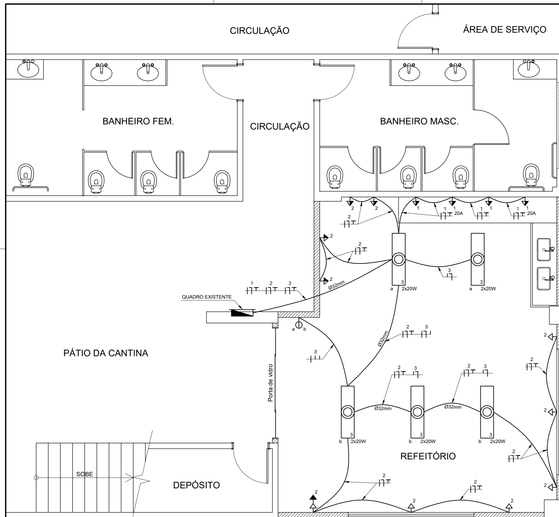
PLANTA BAIXA ESC.: 1/50
