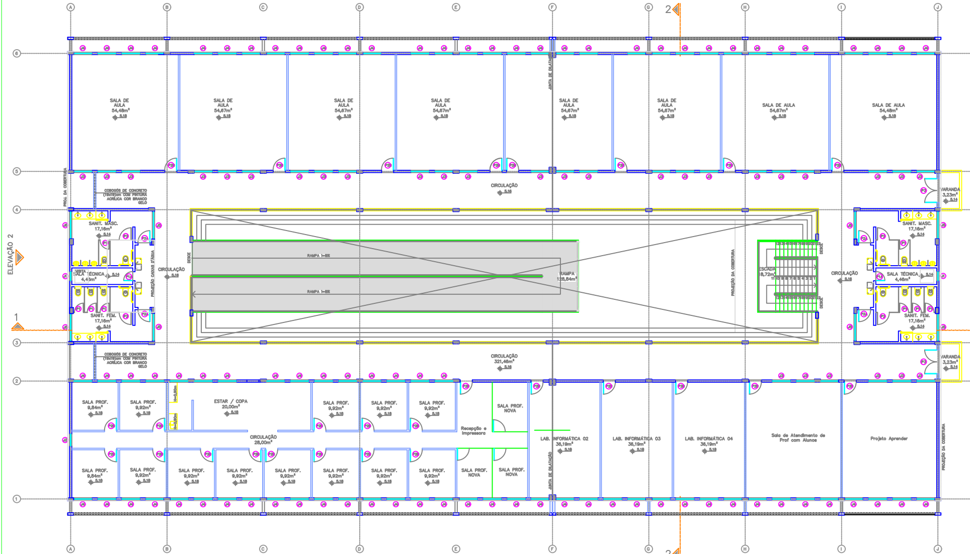
PLANTA BAIXA – PAVIMENTO SUPERIOR Escala 1/75 Área: 1.376,29 m²
