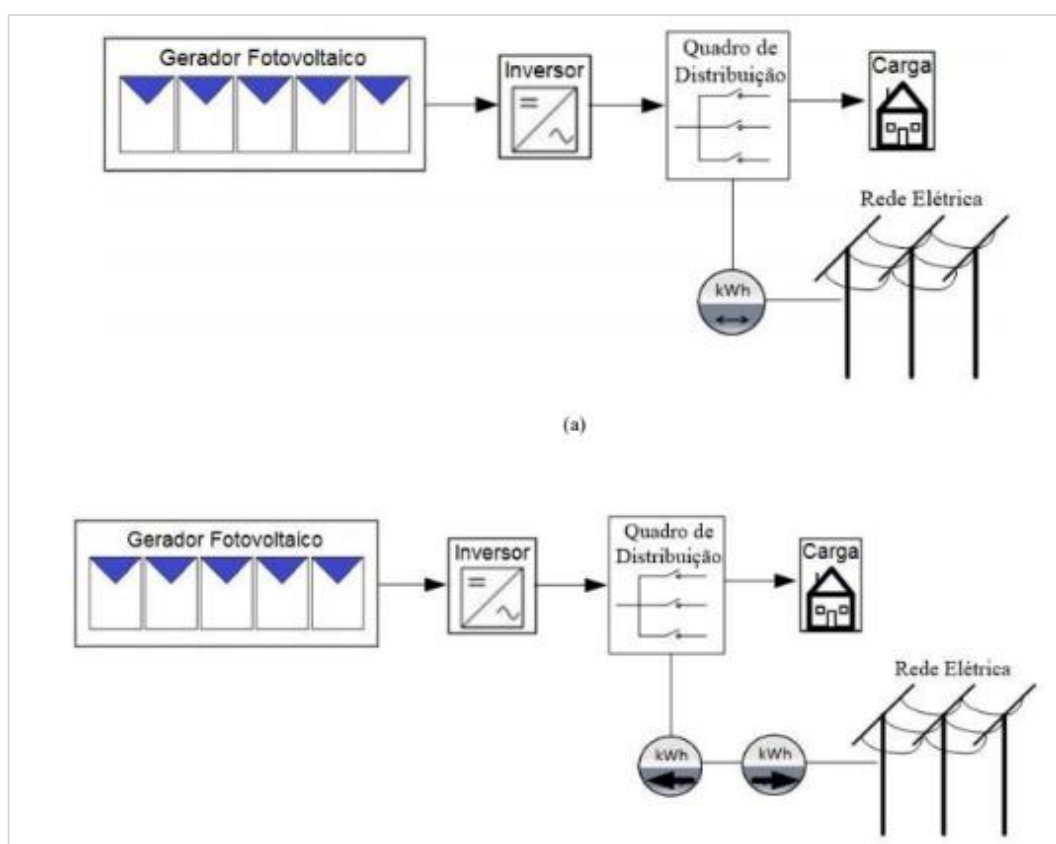
Figura 11 - Medição utilizando um medidor bidirecional e com dois medidores unidirecionais
